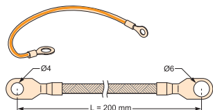
Földelősodrony
