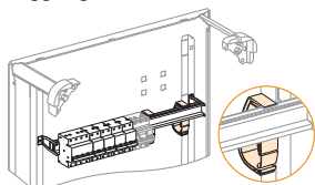
Vízszintes vezetékartó bilincs
