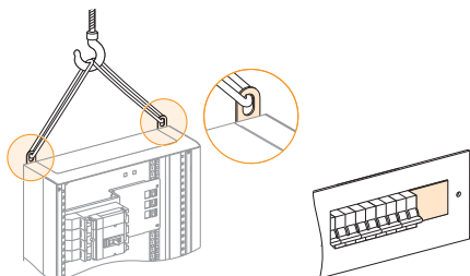
Emelőgyűrű
